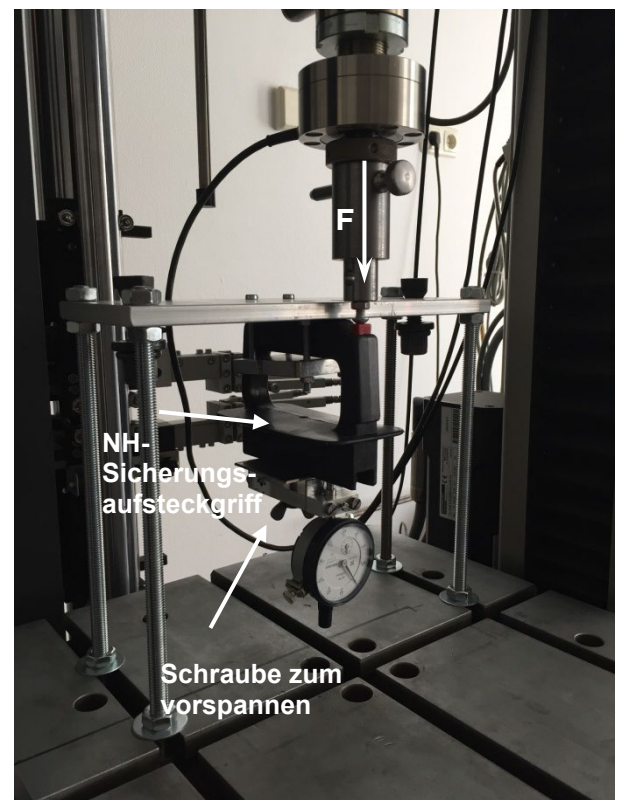
Bild 3: Prüfaufbau Entriegelungskraft
