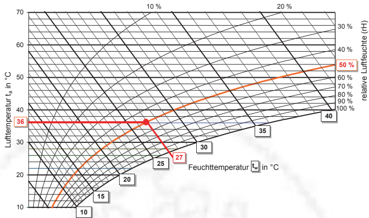
Bild 3: h-x-Diagramm
