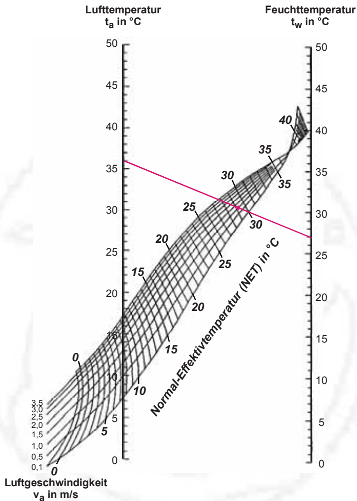
Bild 4: Nomogramm zur Ermittlung der Normal-Effektivtemperatur (NET) nach Yaglou (nach DIN 33403-3 [April 2001])
