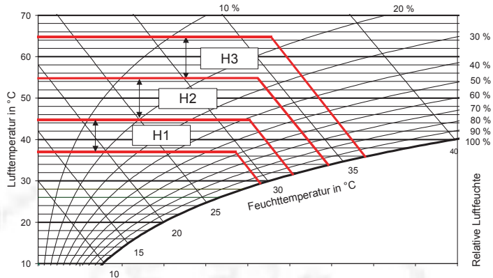
Bild 6: Richtwerte für Entwärmungsphasen bei Hitzearbeit
