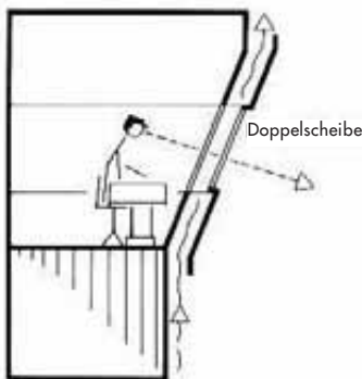
Bild 5: Doppelscheibensystem
